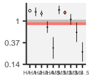
nTreg (1.35e-02)
