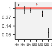
nTconv (4.14e-01)
