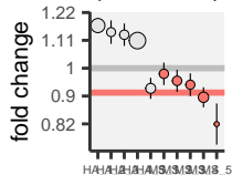
mTconv
