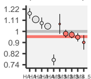
nTreg
