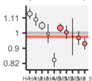
nTconv
